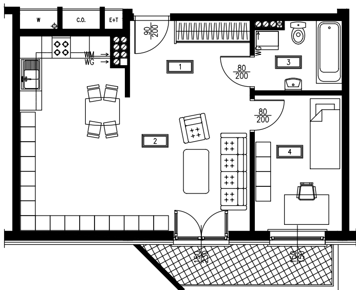
Rzut mieszkania
